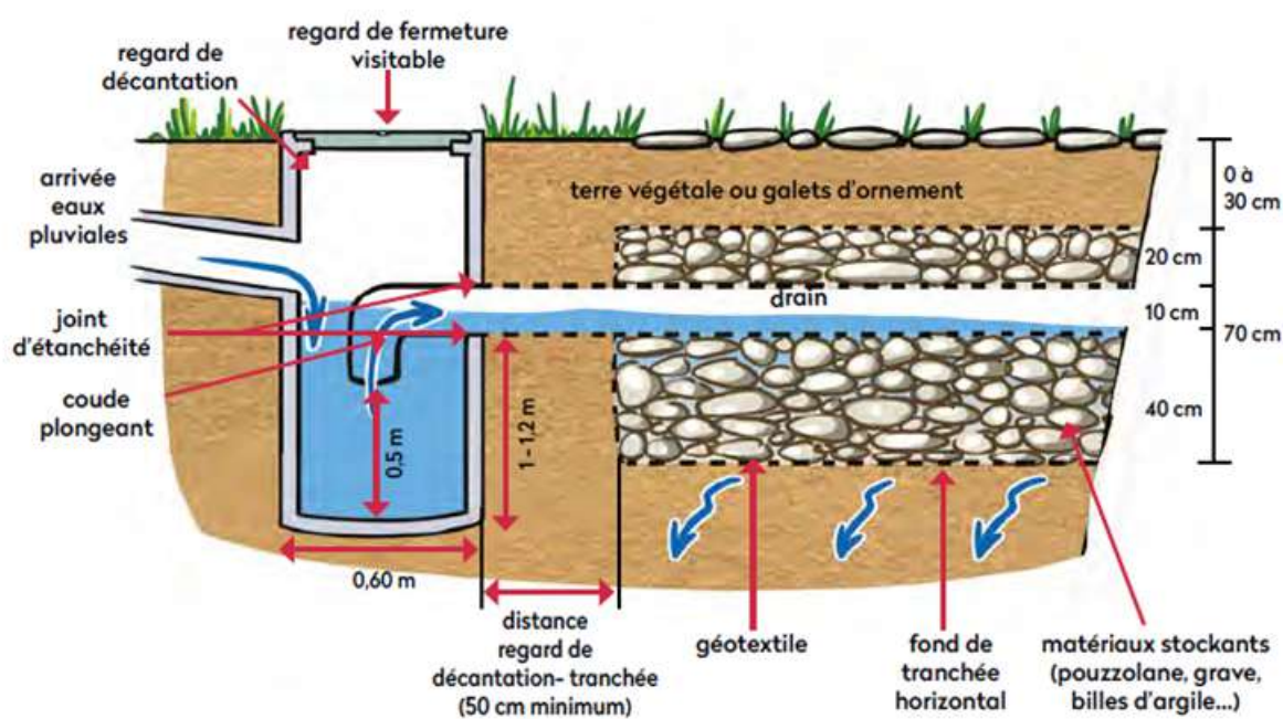
Figure 22 : Coupe longitudinale d'une tranchée
